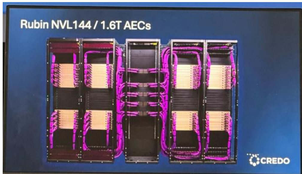
圖 5：Rubin NVL144 透過 72 條 AEC 實現後端互連、18 條用於前端連接
